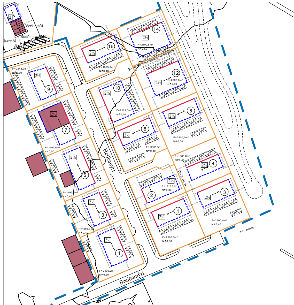
Deiliskipulag fyrir breytingu - mkv. 1:2.000
