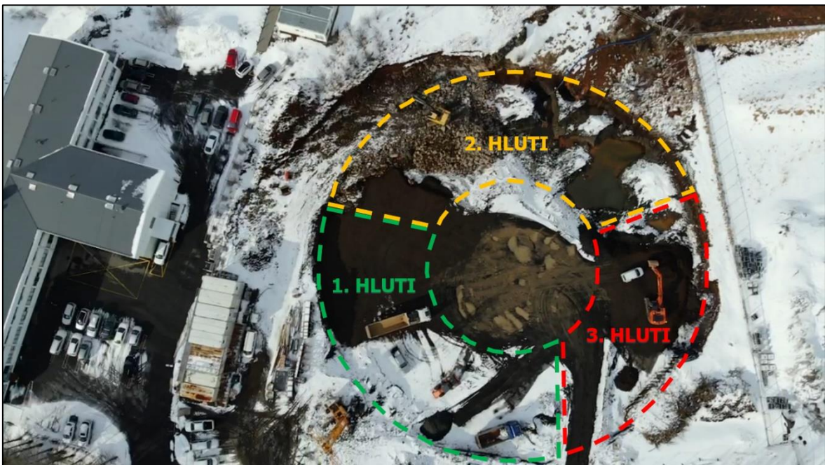
Myndin hér að ofan sýnir nokkurn veginn hvernig fyrirhugað er að skipta púðanum í þrjá hluta, með það að markmiði að hefja vinnu við uppslátt sökkla sem fyrst. Ljósmynd: Birgir Leó Ólafsson, Mannvit.
