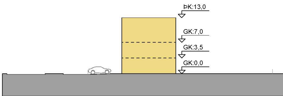
Mynd 28: F2 - Sneiðing 1:500
