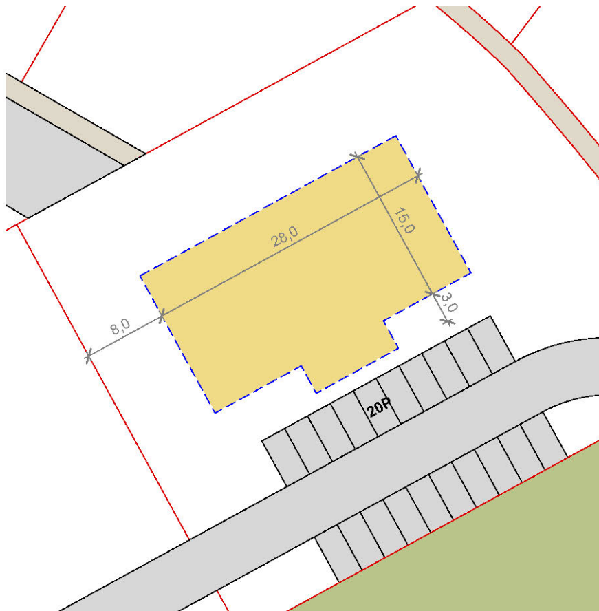
Mynd 36: F5 - Skilmálateikning 1:500
