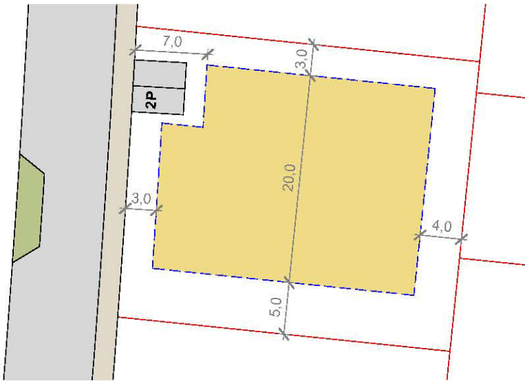
Mynd 12: E2 - Skilmálateikning 1:500
