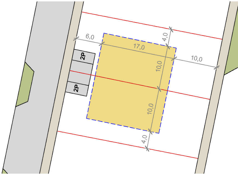
Mynd 15: P1 - Skilmálateikning 1:500
