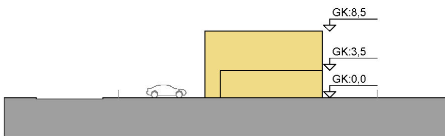
Mynd 22: K1 - Sneiðing 1:500
