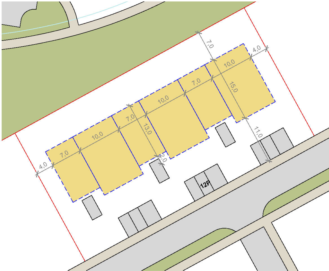
Mynd 21: K1 - Skilmálateikning 1:500
