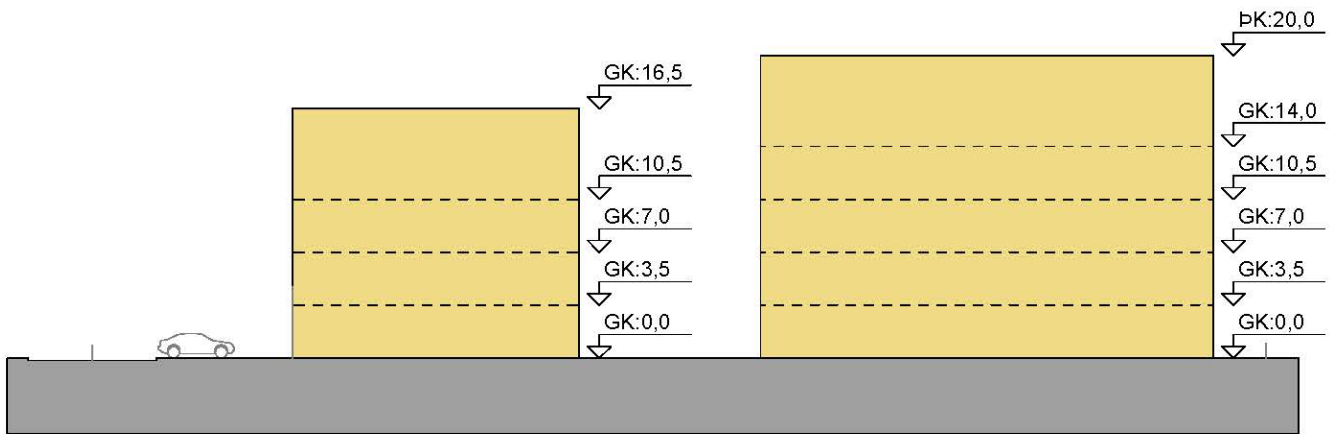
Mynd 34: F4 - Sneiðing 1:500
