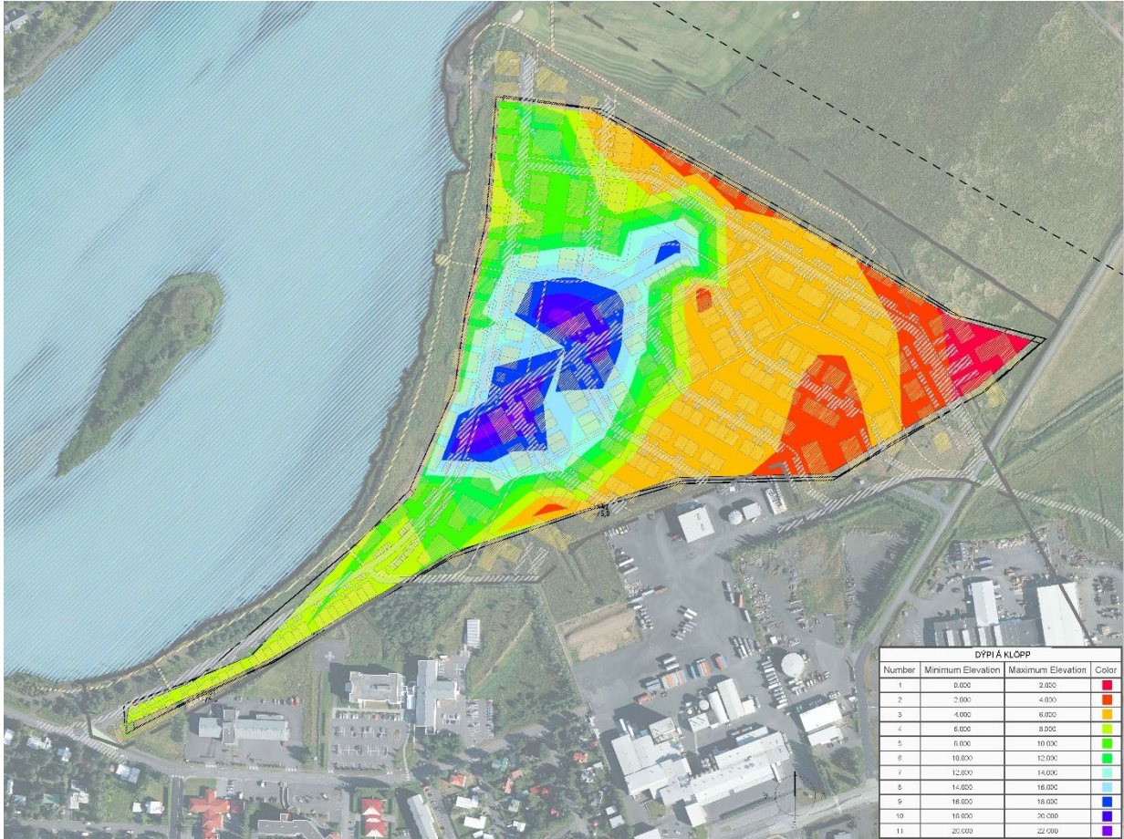
Mynd 3: Úr skýrslu VSÓ. Dýpi á klöpp
