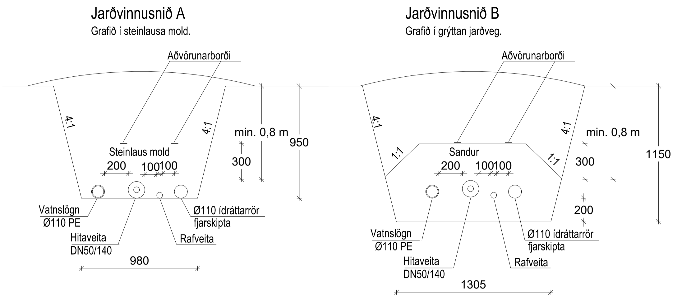
SNIÐ 1:20
