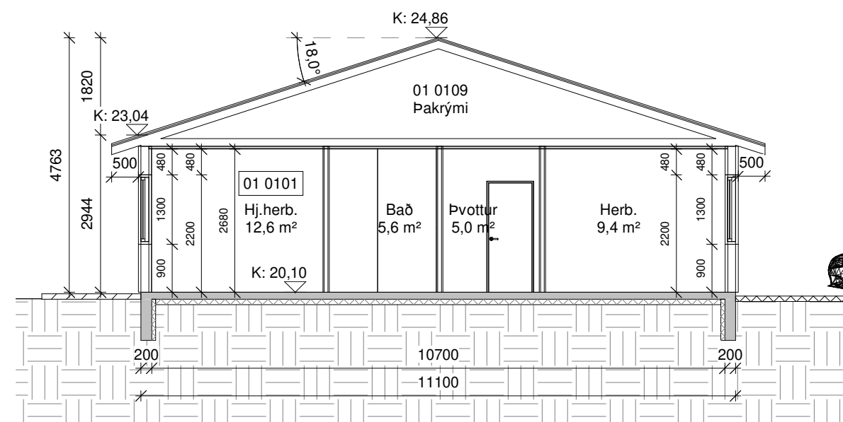
Snið A-A
