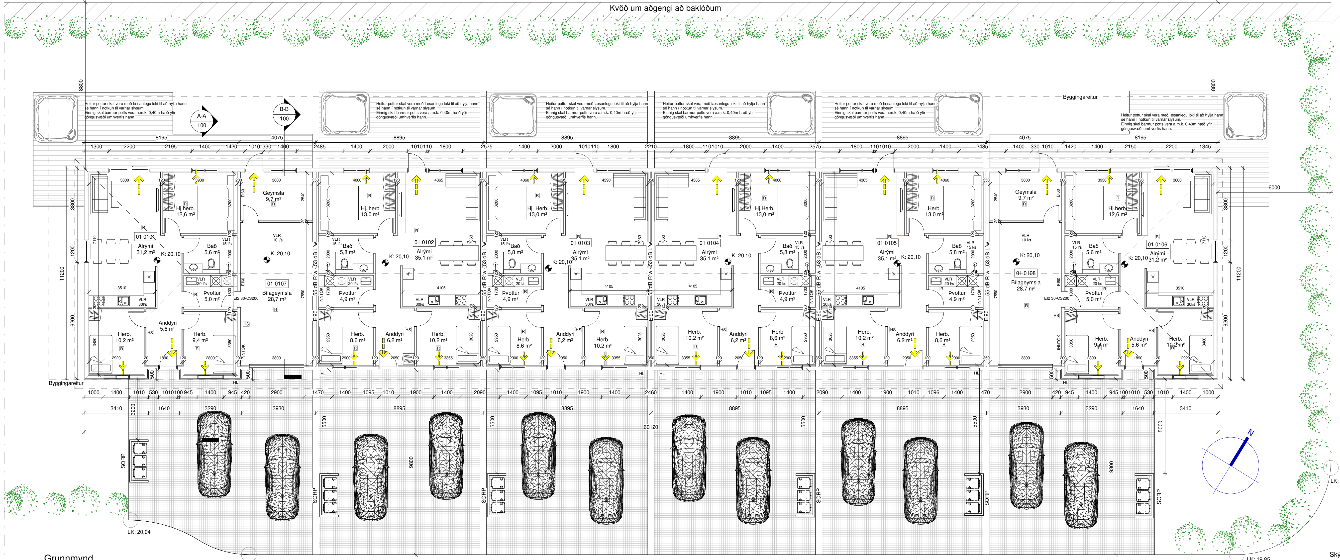
Grunnmynd
