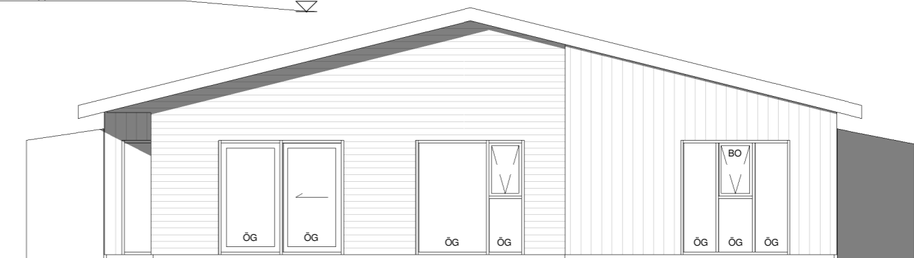
Suðaustur 1 : 100
