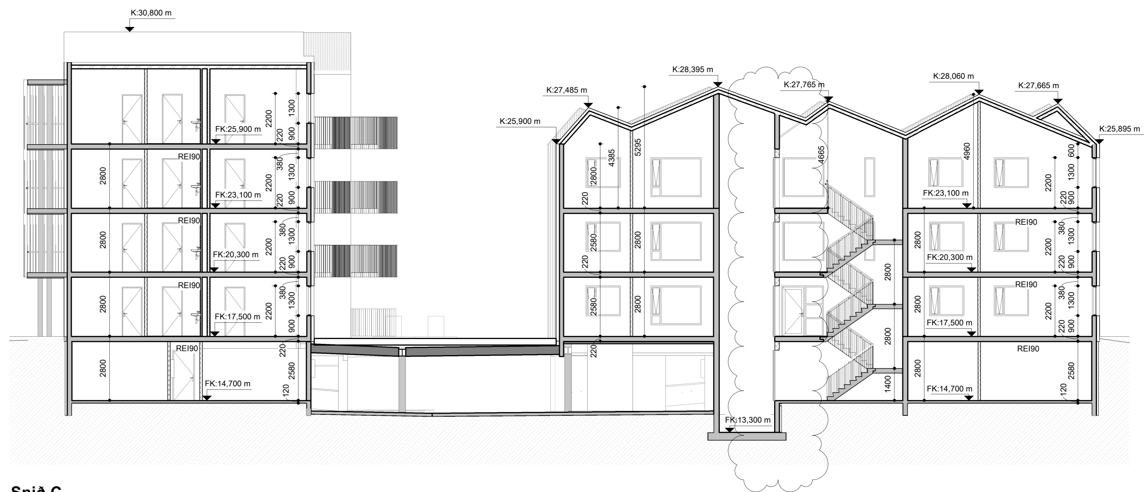
Snið C mkv: 1 : 100
