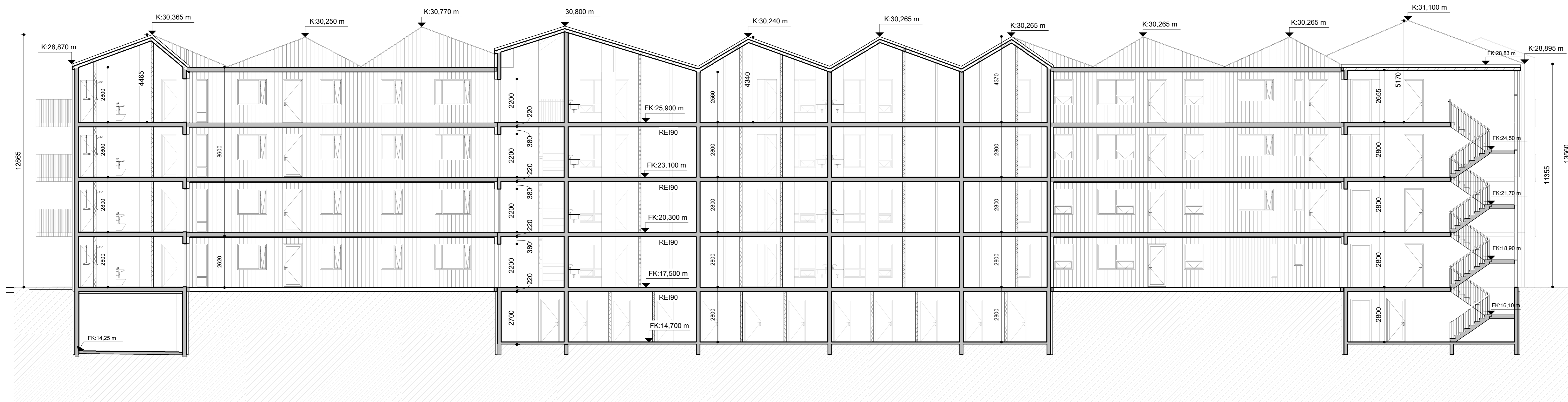
Snið B mkv: 1 : 100
